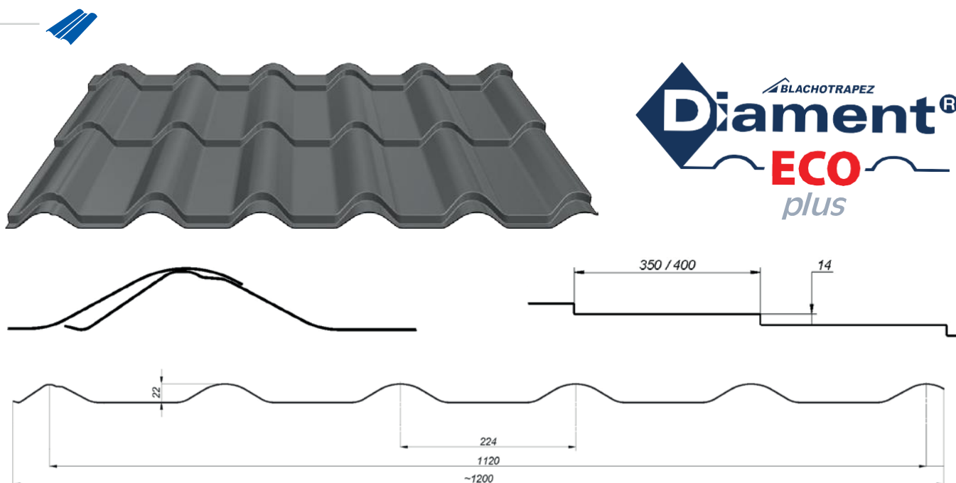
Diamant Eco Plus - Méretek, Keresztmetszet és hosszmetset.
